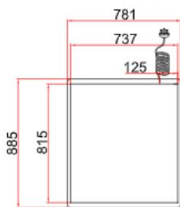
PLAIN 顶视图
